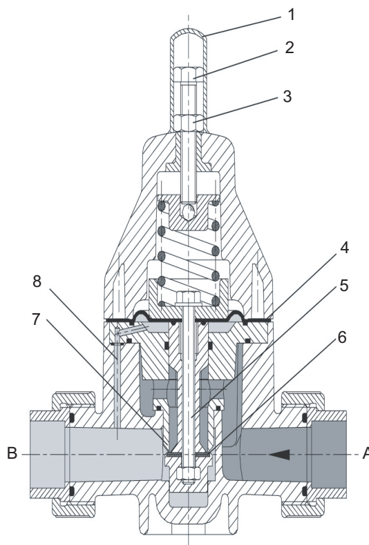
Рис. 2 Конструкция DMV 755
