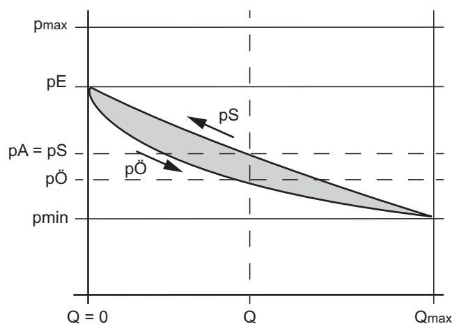
Рис. 13 Рабочие характеристики
