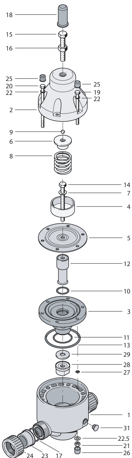
Рис. 6 Чертеж DMV 755
