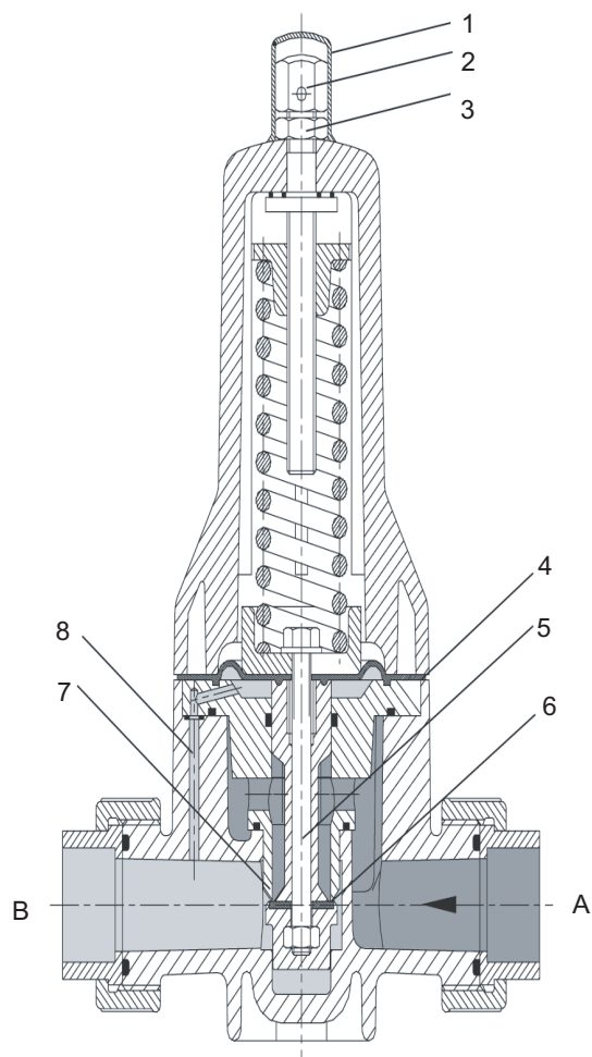
Рис. 3 Конструкция DMV 765
