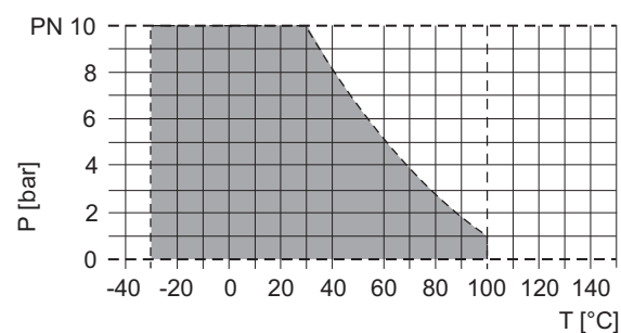
Рис. 10 Предельные значения давления и температуры PVDF
