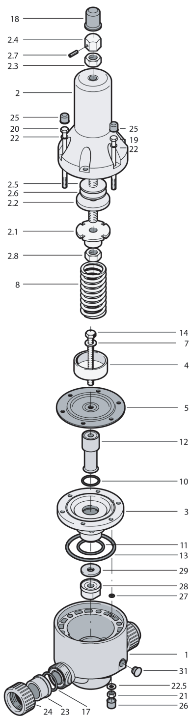
Рис. 7 Чертеж DMV 765
