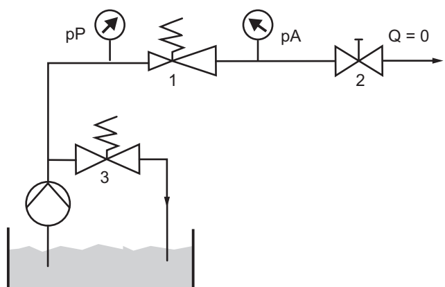
Рис. 12 Пример 2. Вторичное давление – система закрыта
