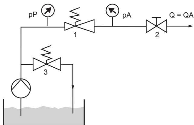
Рис. 11 Пример 1. Вторичное давление – динамический поток в системе
