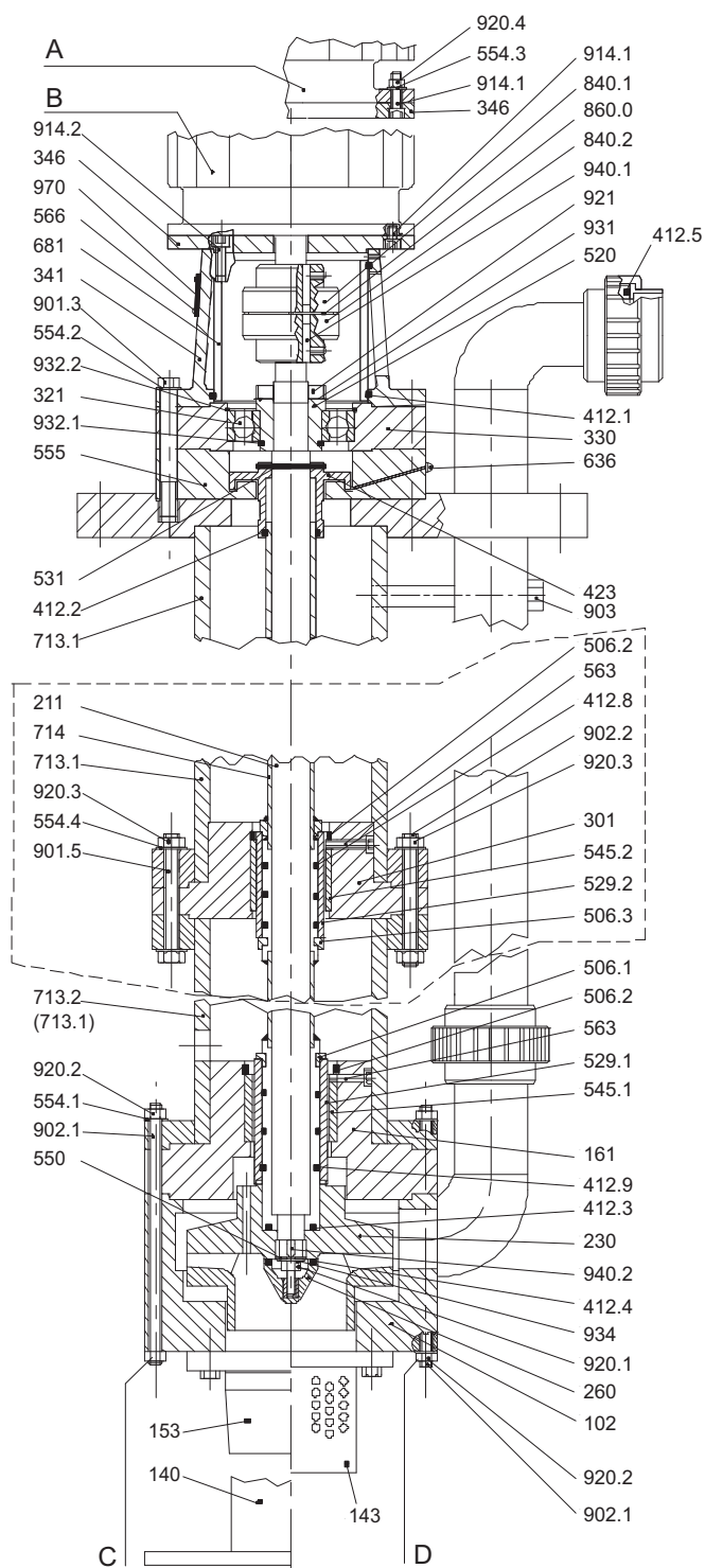
Рис. 4 Запасные детали ET 32-160 до 80-250, исполнение с лабиринтным уплотнением
