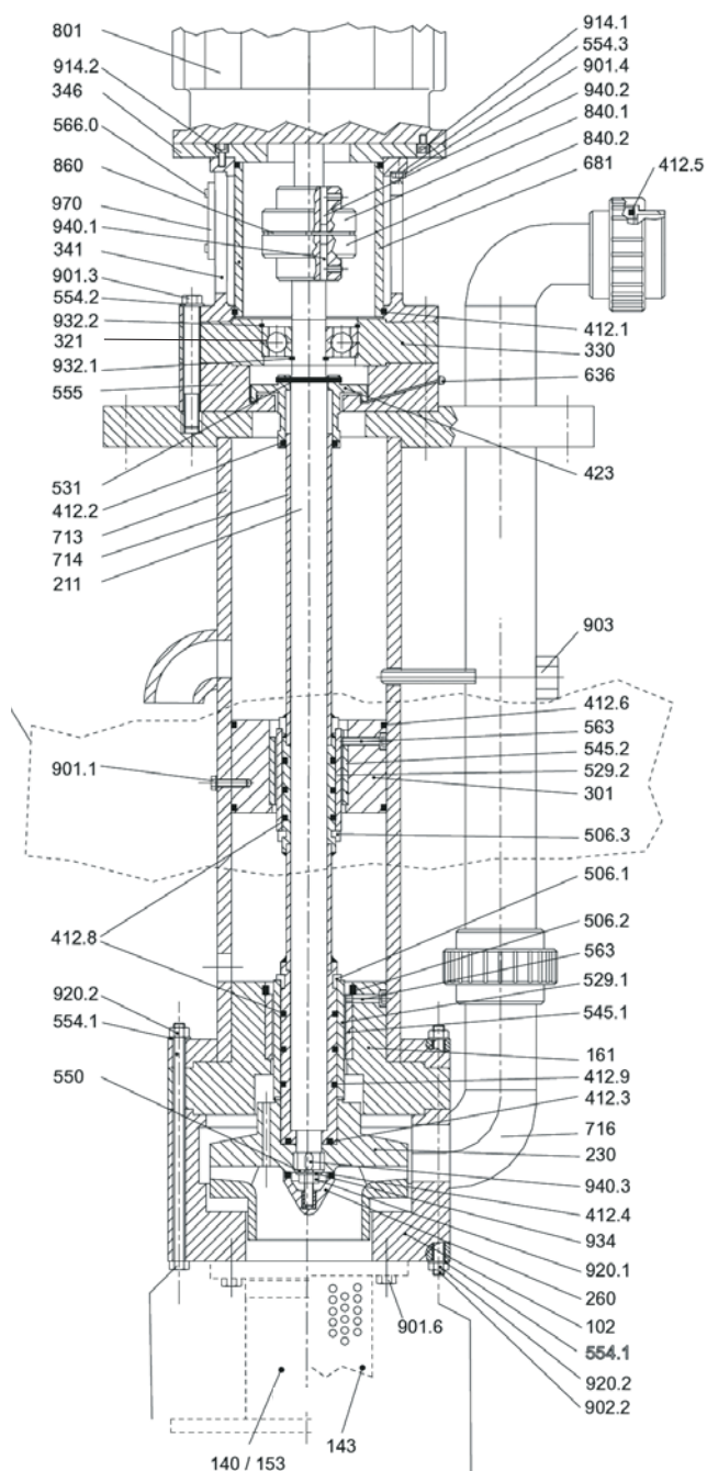
Рис. 3 Запасные детали ЕТ 15–80 до 40–125, исполнение с лабиринтным уплотнением
