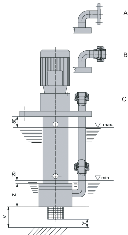
Рис. 5 Монтажные размеры и уровни заполнения
