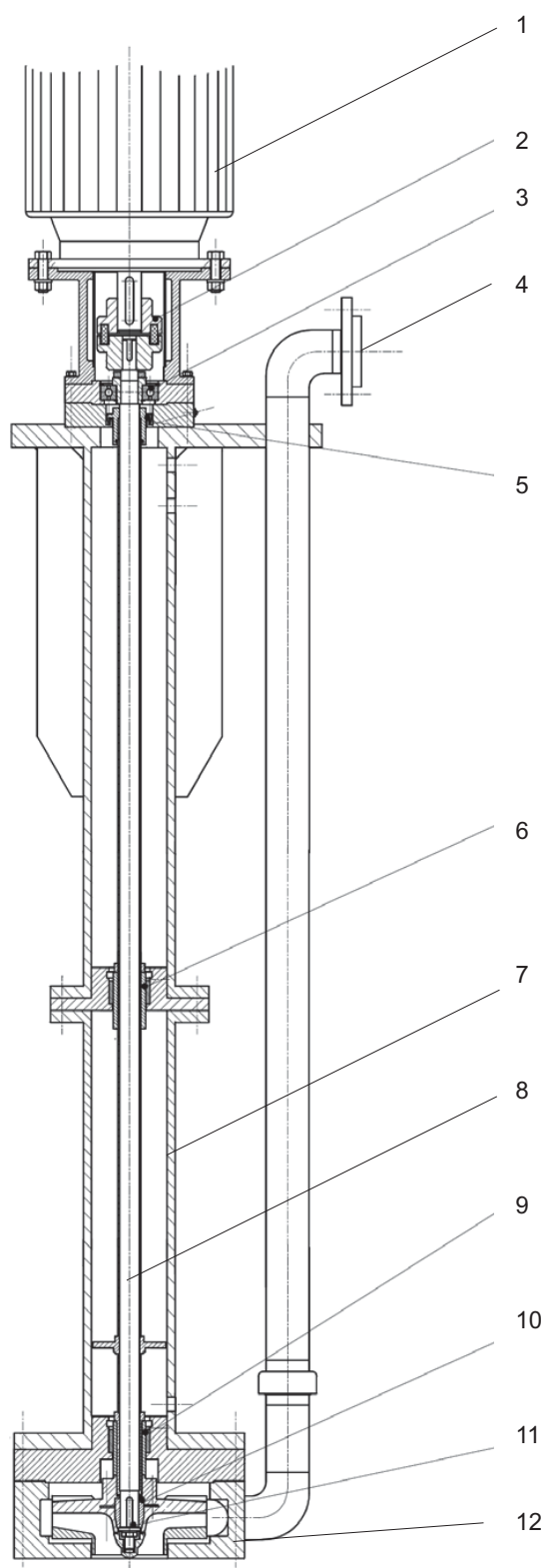
Рис. 2 Конструкция
