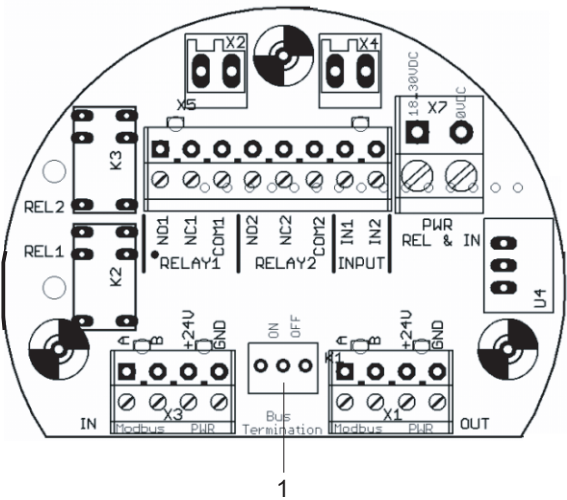
Рис. 6 Схема подключений Modbus RTU
