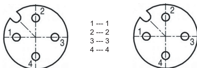
Рис. 7 Разводка контактов, вариант Flex
