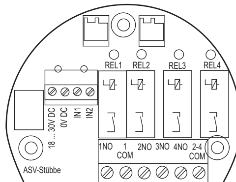
Рис. 8 Схема соединений реле
