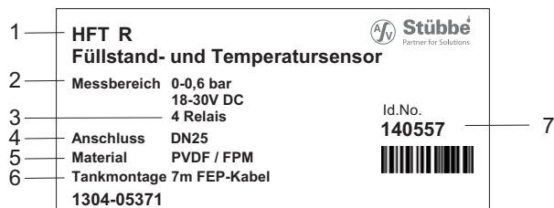
Рис. 1 Заводская табличка (пример)
