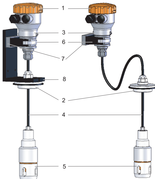
Рис. 3 Конструкция корпуса и датчика Flex
