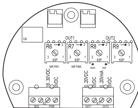
Рис. 7 Настройка потенциометра
