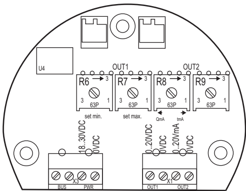
Рис. 9 Схема соединений тока
