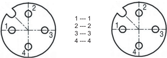
Рис. 10 Разводка контактов, вариант Flex
