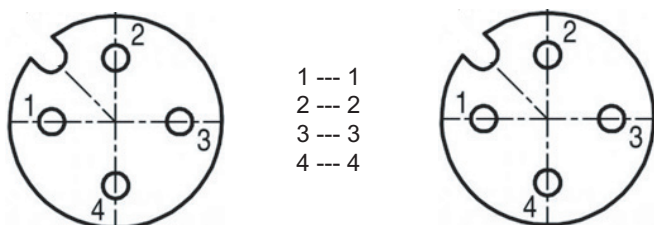
Рис. 9 Разводка контактов, вариант Flex
