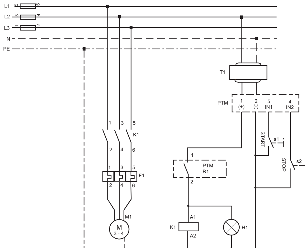
F1 Реле защиты двигателя H1 Контрольная лампа насоса K1 Контроллер для управления электродвигателем M1 Двигатель насоса s1 Кнопка пуска s2 Кнопка остановки T1 Сетевой блок питания 24 В пост. тока
