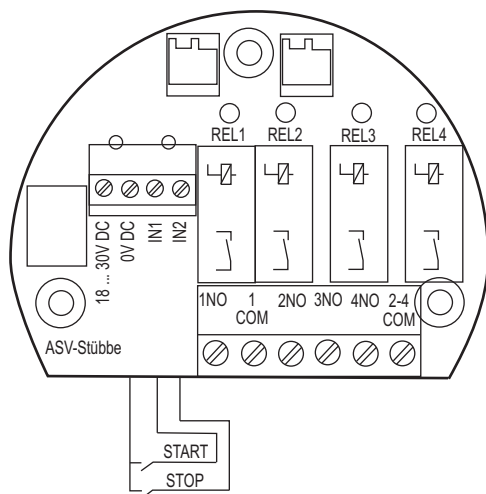
Рис. 8 Схема соединений
