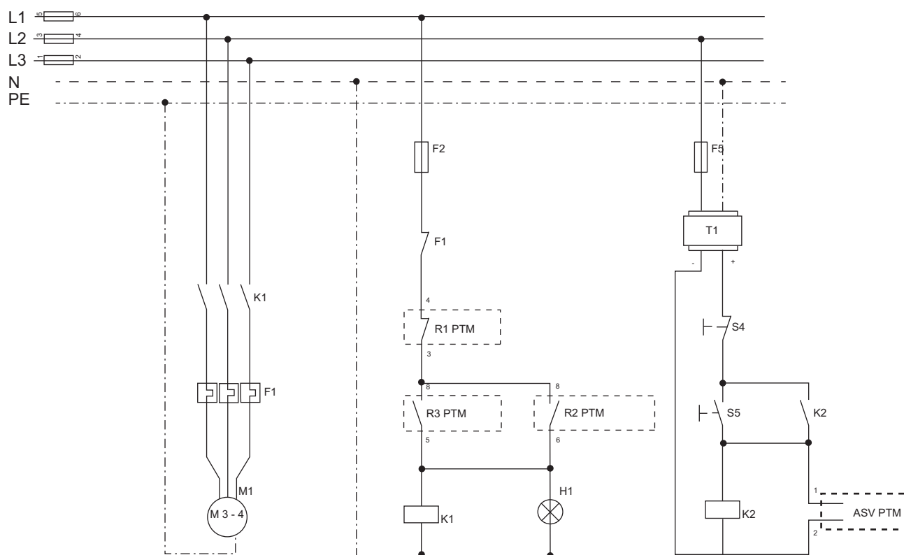
Рис. 7 Схема соединений контроля слишком высокого и слишком низкого давления
