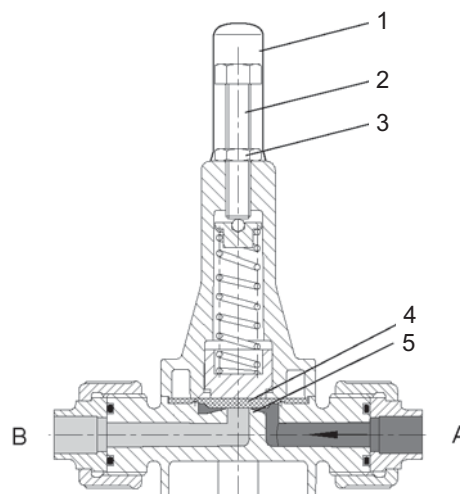
Рис. 2 Конструкция DHV 718, DN8
