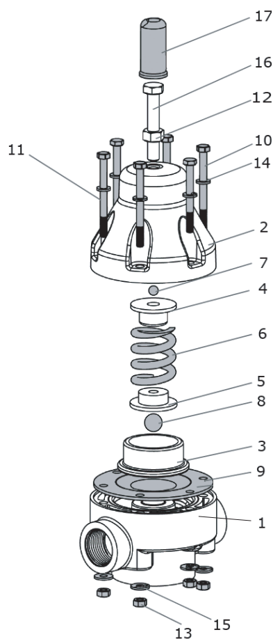
Рис. 7 Чертеж DHV 718, DN 10–DN 50
