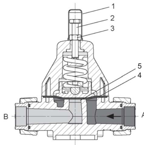
Рис. 3 Конструкция DHV 718, DN 10–DN 15
