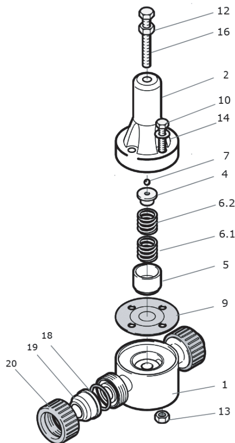
Рис. 6 Чертеж DHV 718, DN 8
