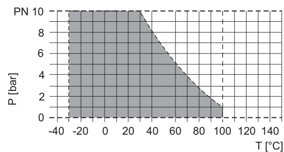
Рис. 10 Предельные значения давления и температуры PVDF, PTFE, V4A
